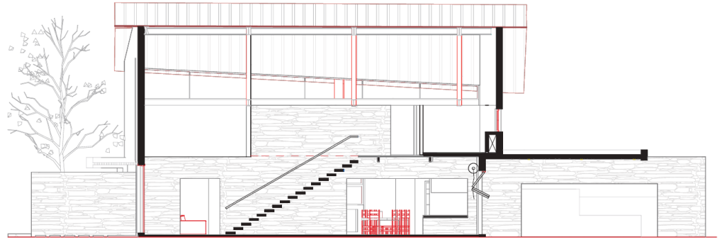
section a-a 1:100
